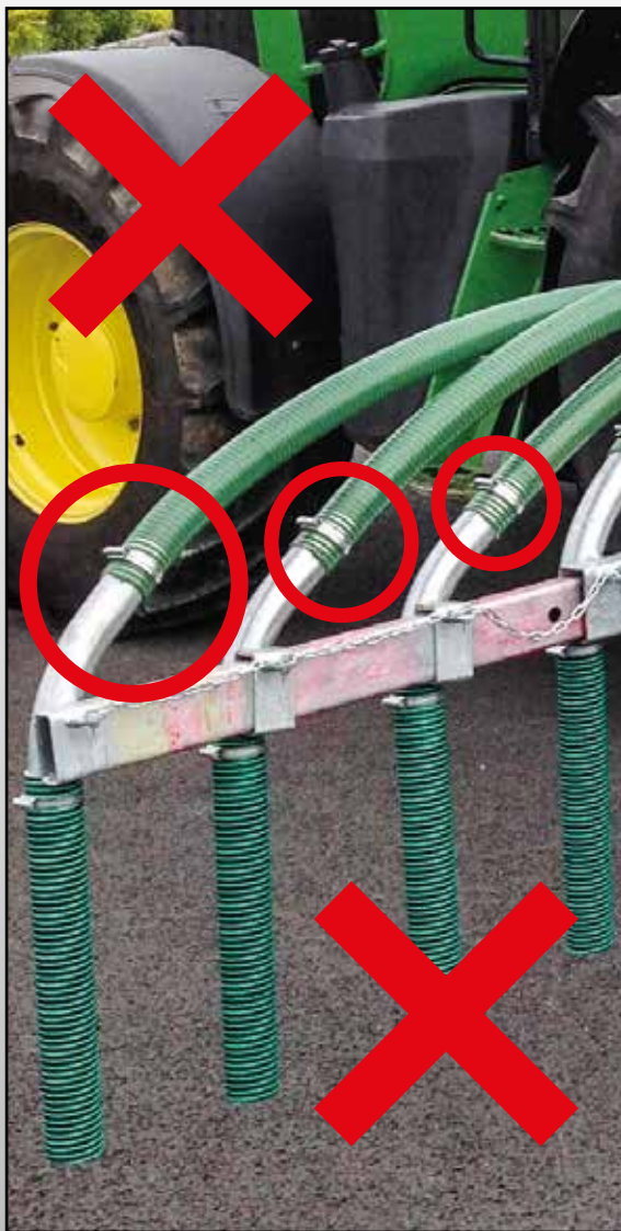
50 mm slanger m/ innvendige stålør som gir blokkeringer.
